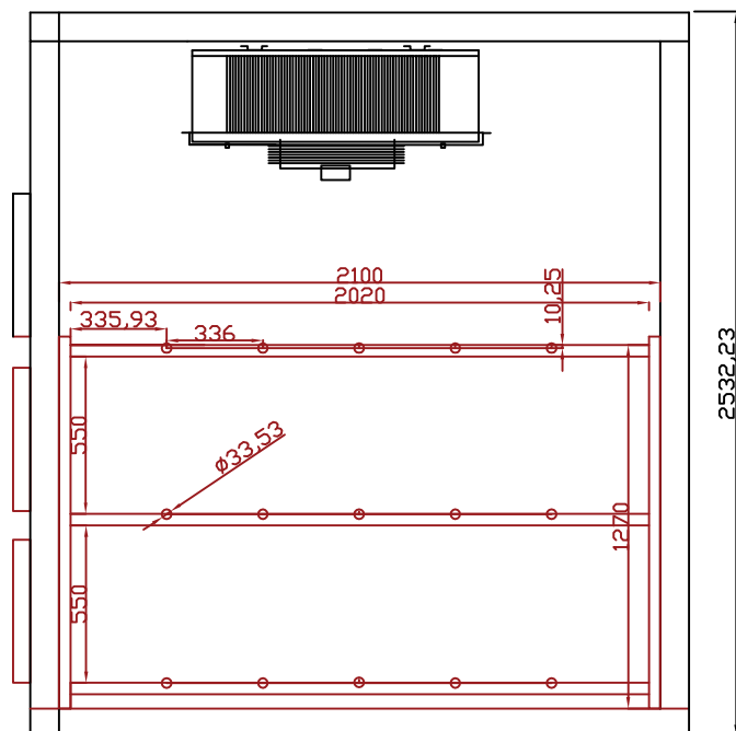
Pogled sa bočne strane sa merama klizača unutar komore
