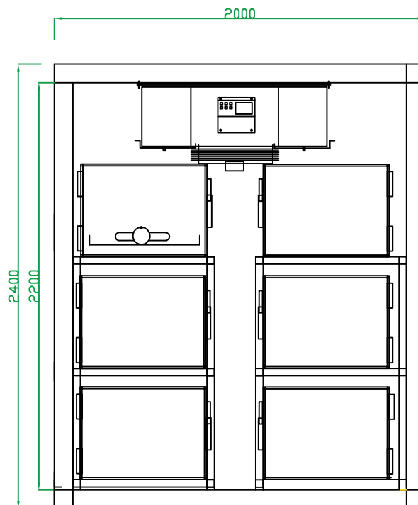
pogled na komoru od prednje strane u preseku sa nosačima, isparivačem rocesorom
